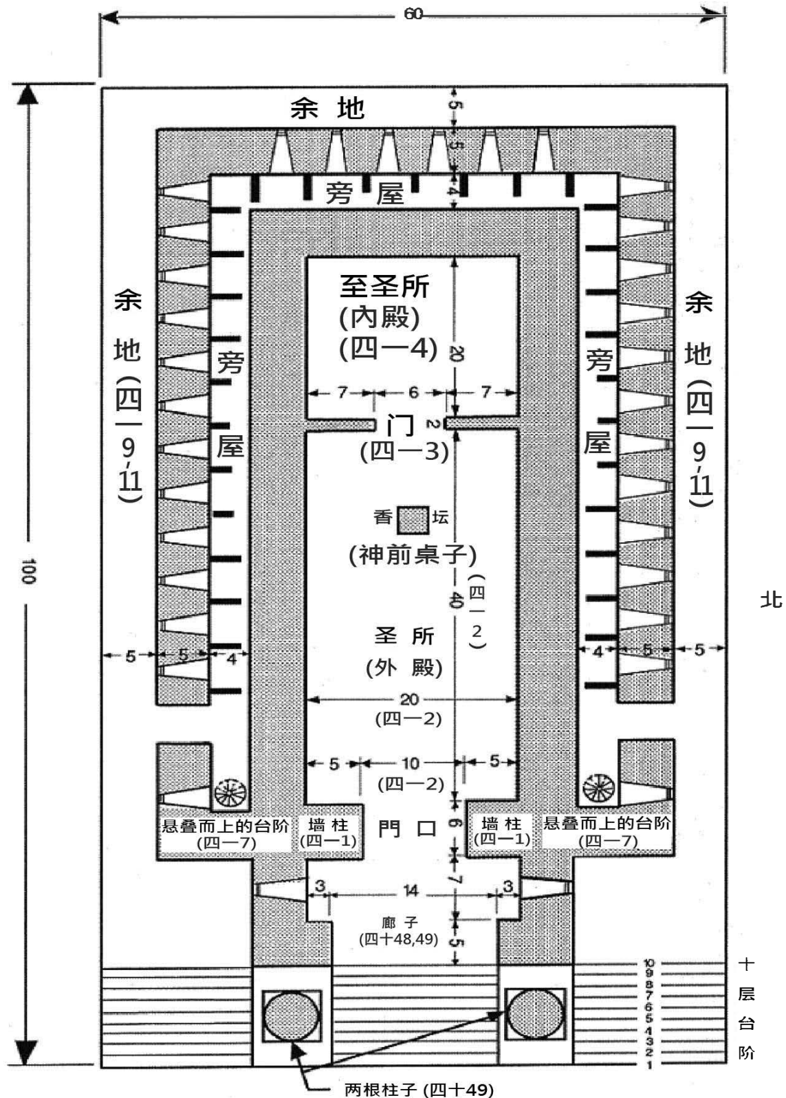
第四图：圣殿平面图
