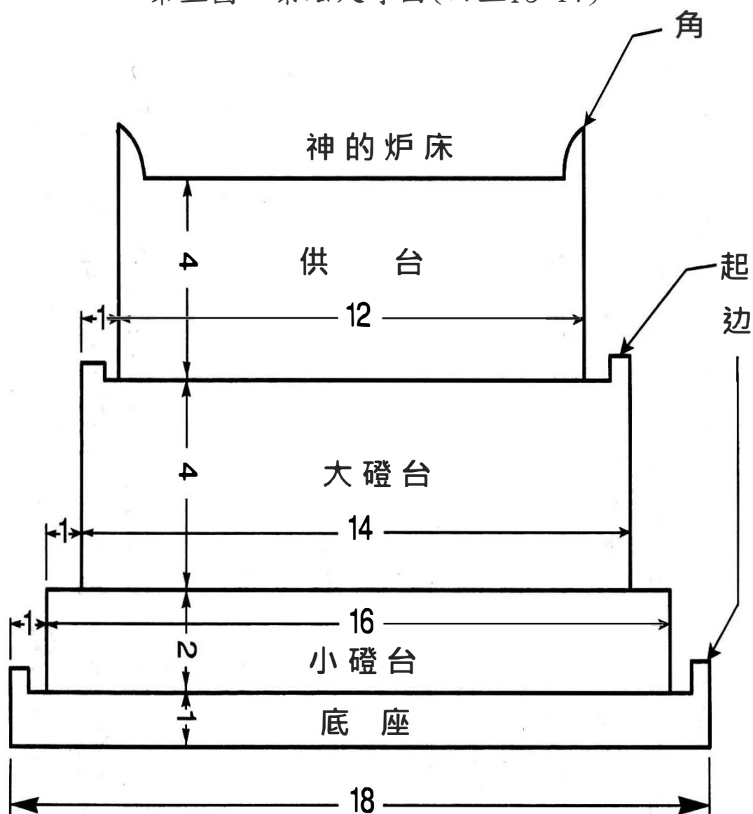
第三图：祭坛尺寸图(四三13~17)
