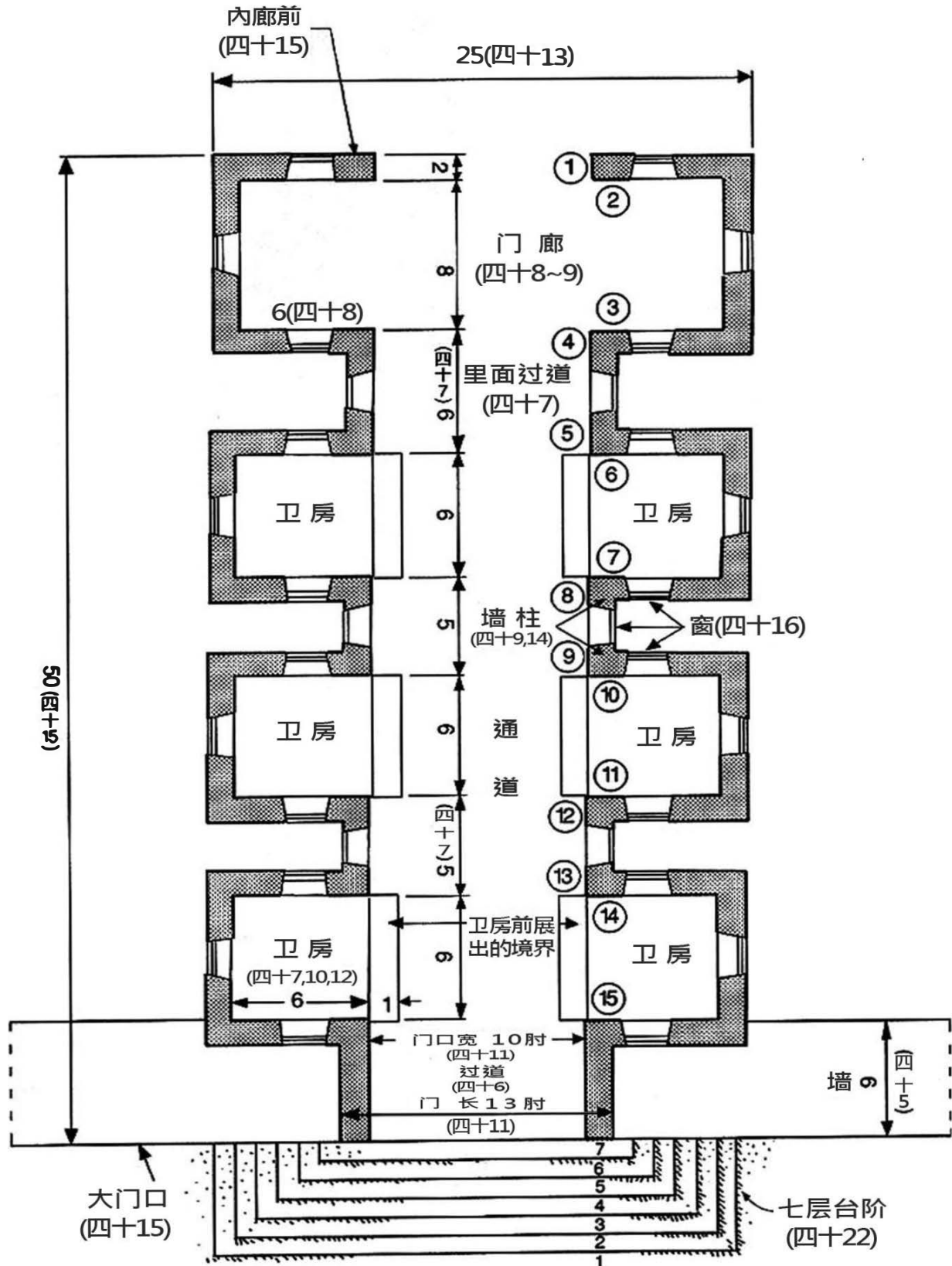
第二图：门洞平面图
